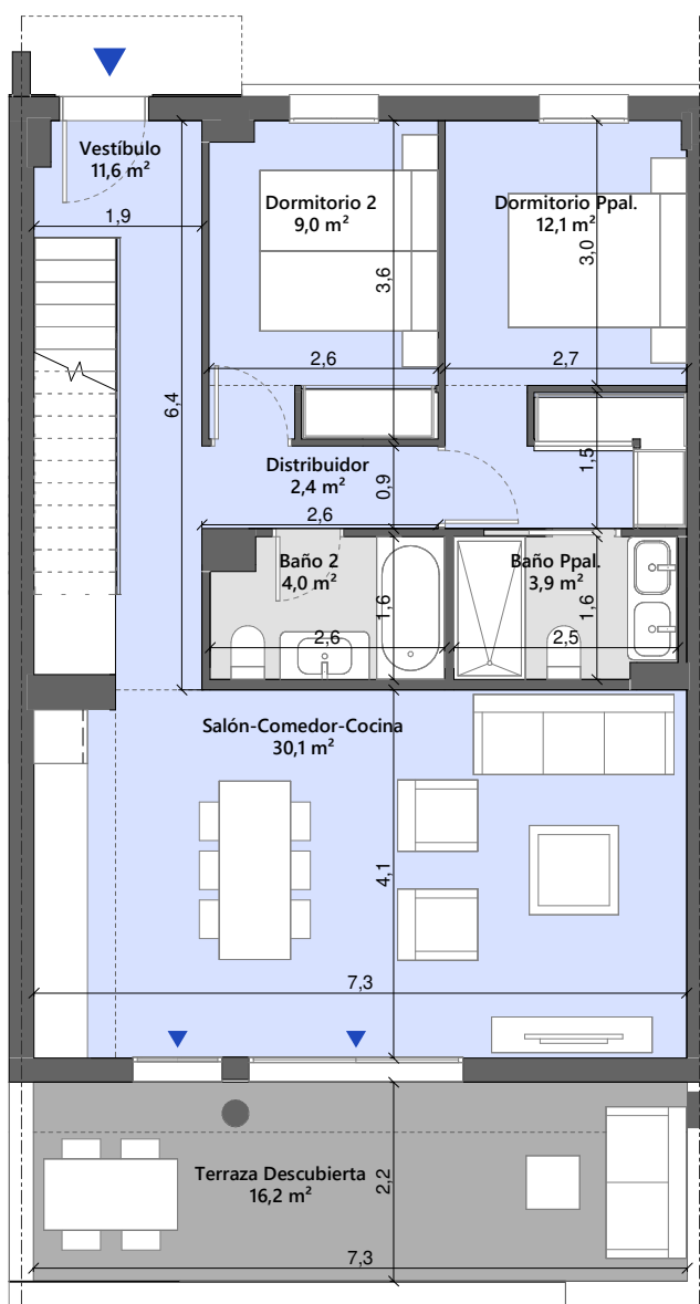
PLANTA BAJA
